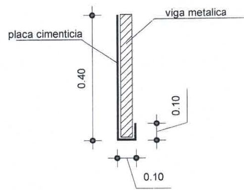
DETALHE REVESTIMENTO DA PLACA CIMENTICIA SEM ESCALA
