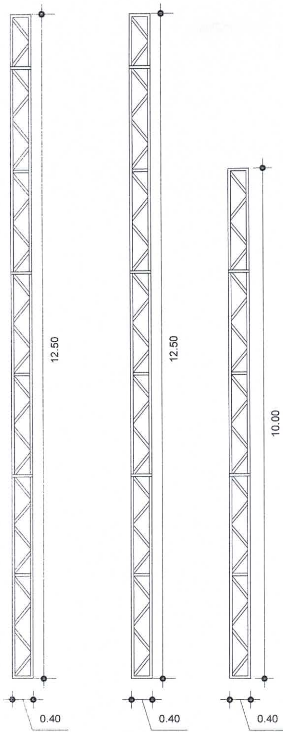
DETALHE DAS TESOURA METALICAS ESCALA.....1/75
